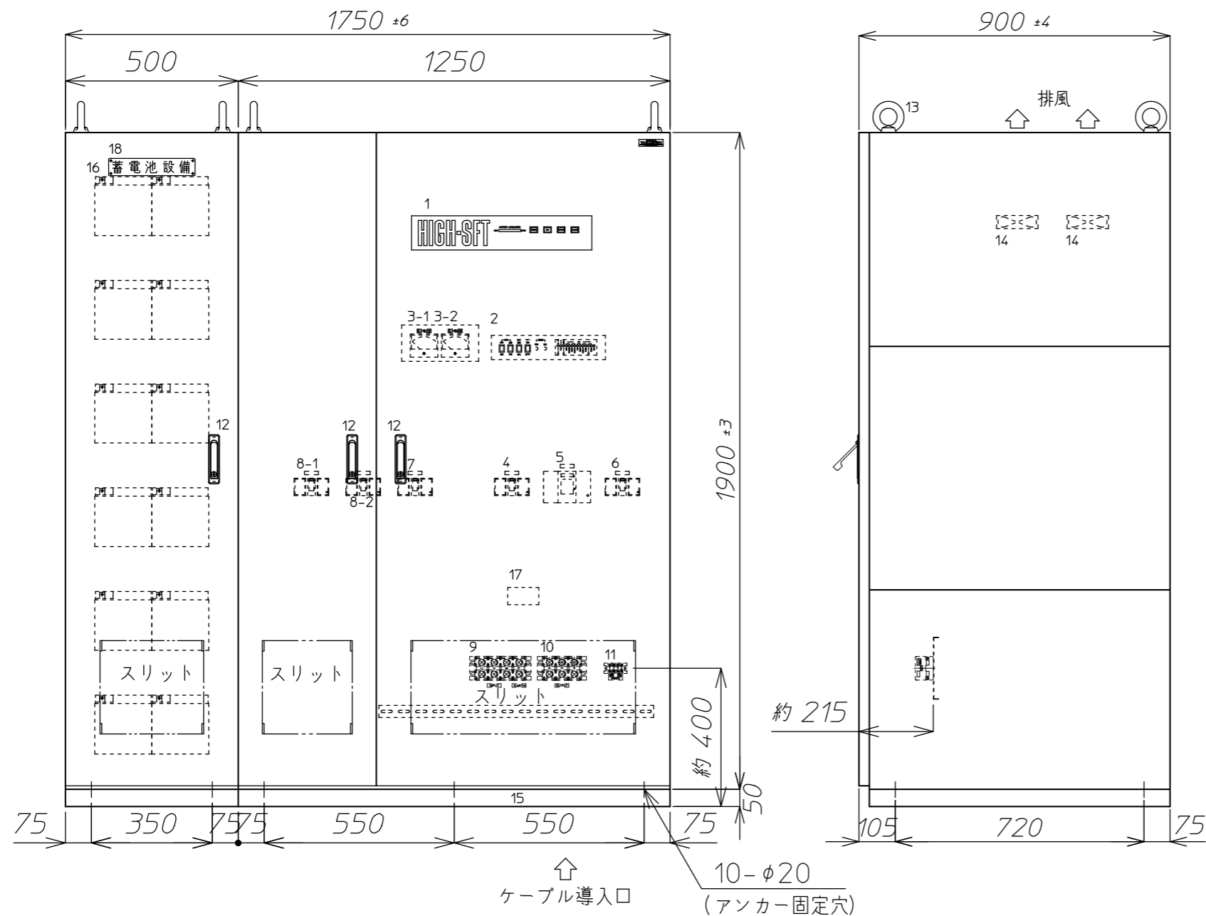
正面図
