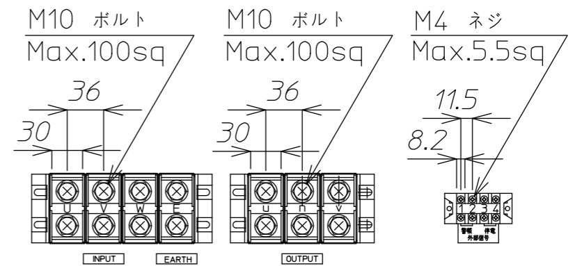
端子詳細図
