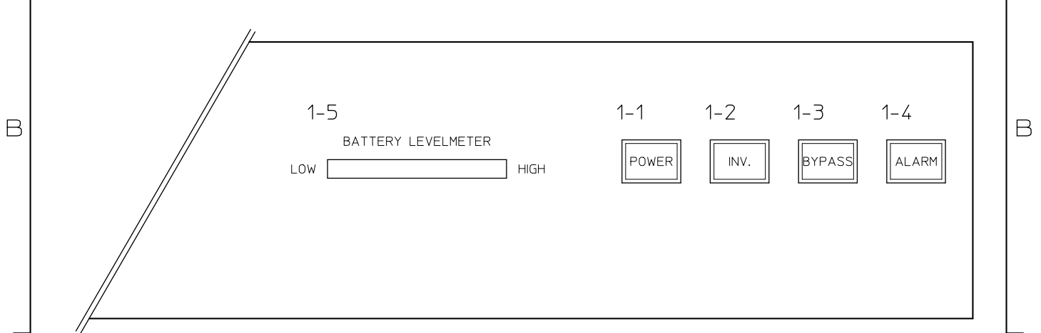
パネル部詳細
