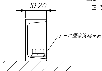
A-A矢視図
