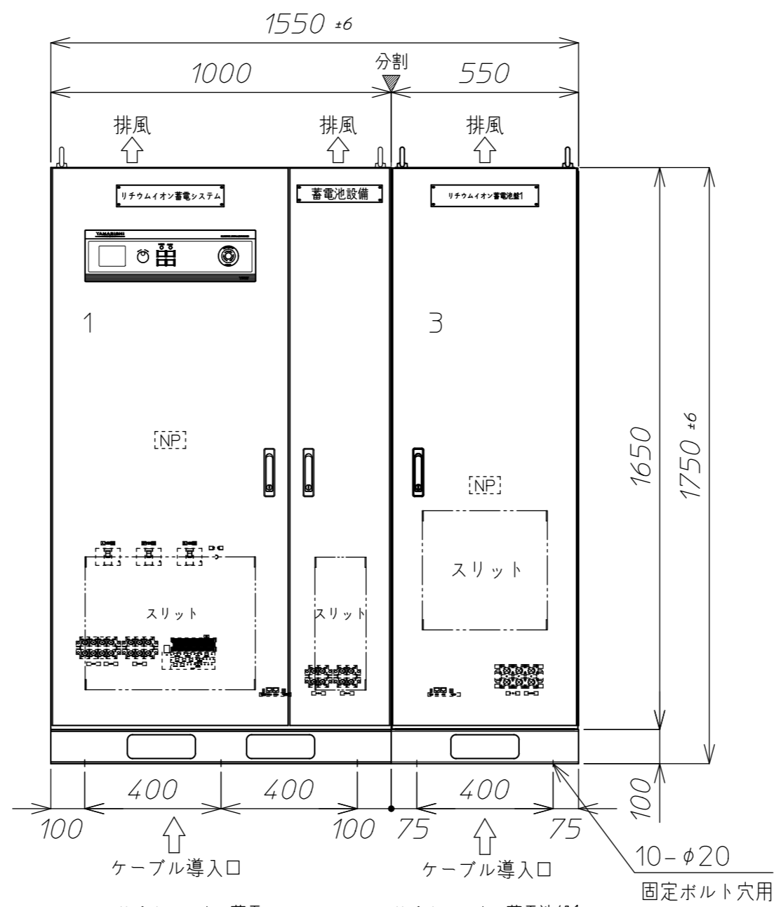
正面
