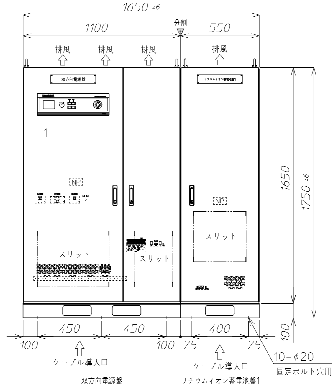
正面
