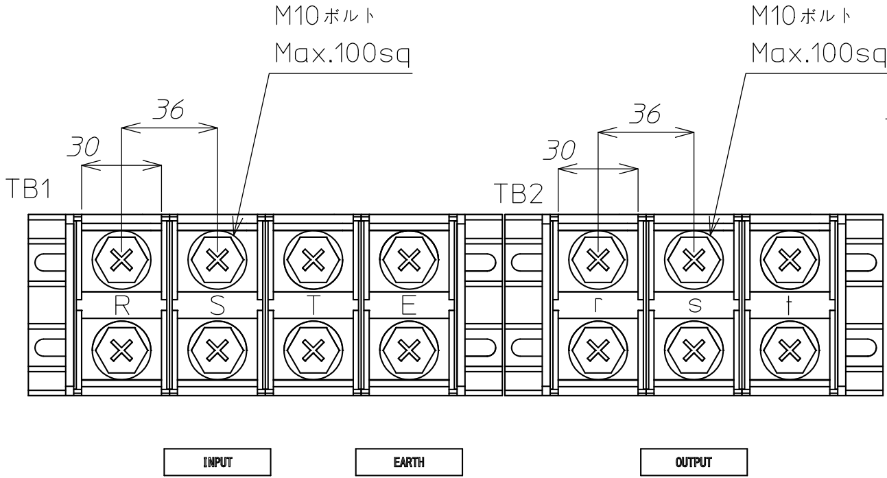
正面端子部
