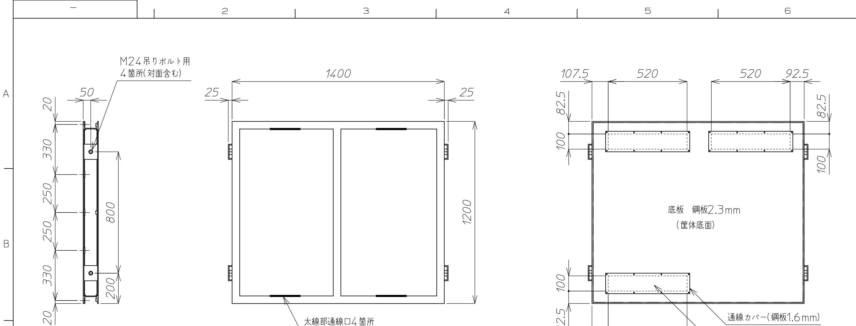
左側面
