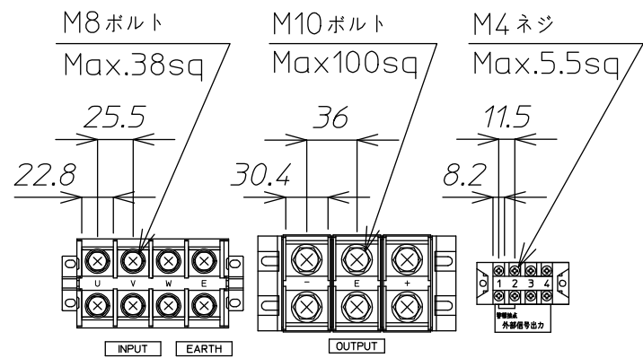
端子詳細図
