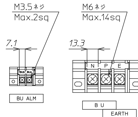
端子詳細図
